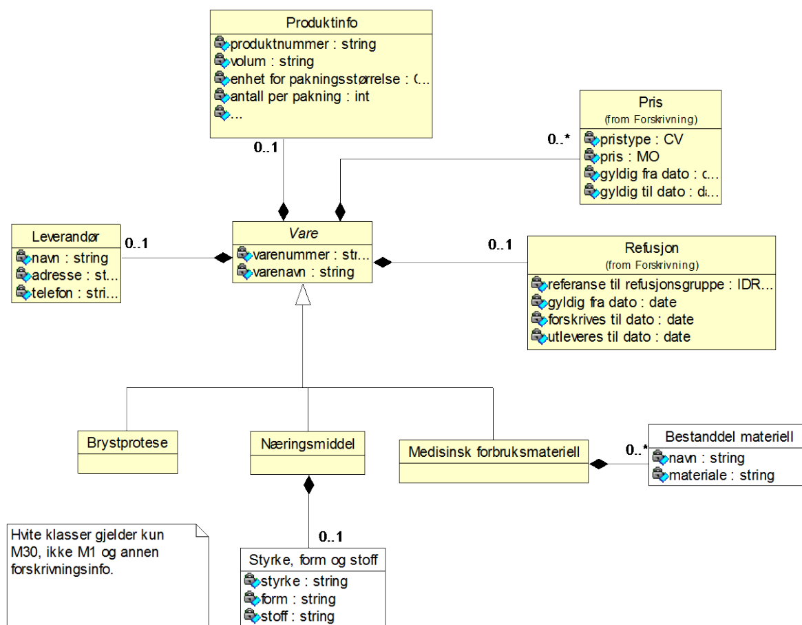
Diagram: Handelsvare
