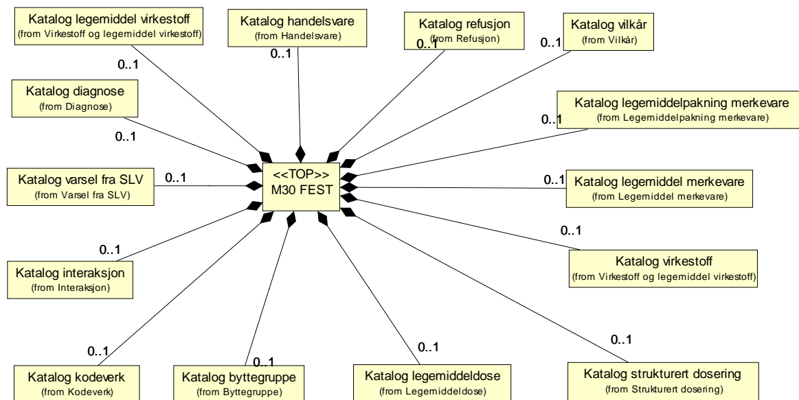
Diagram: Kataloger
