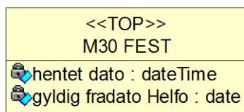
Diagram: Kataloger
