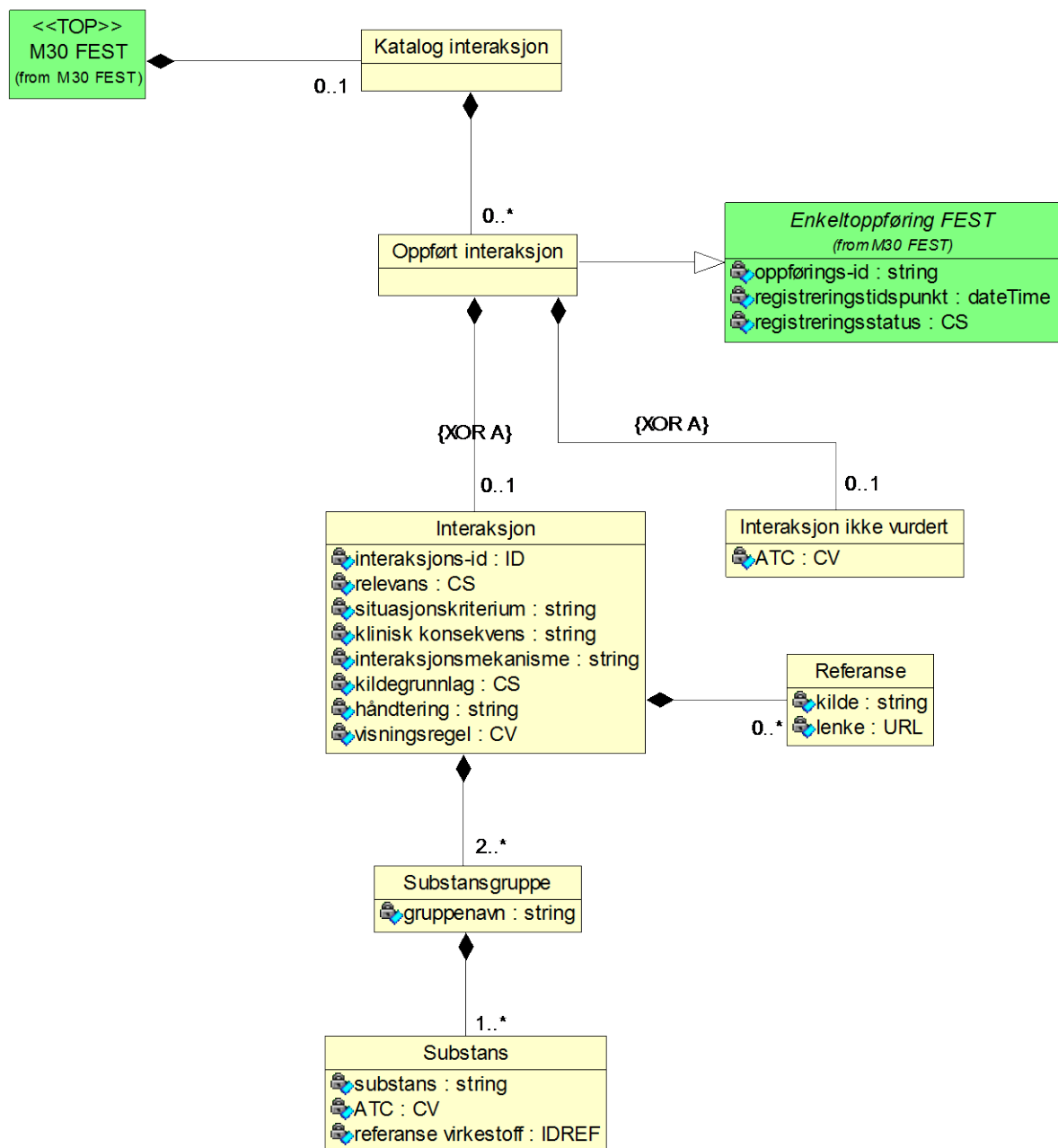
Diagram: Interaksjon
