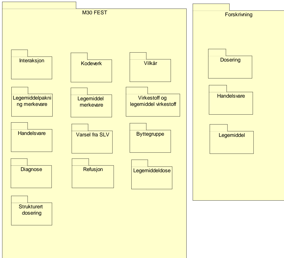
Figur 1 Pakkeoversikt
