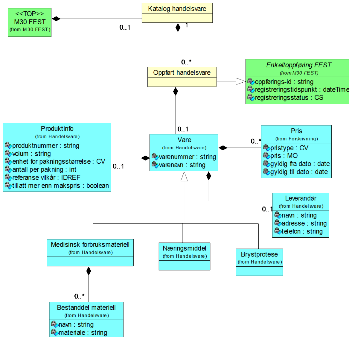
Diagram: Handelsvare
