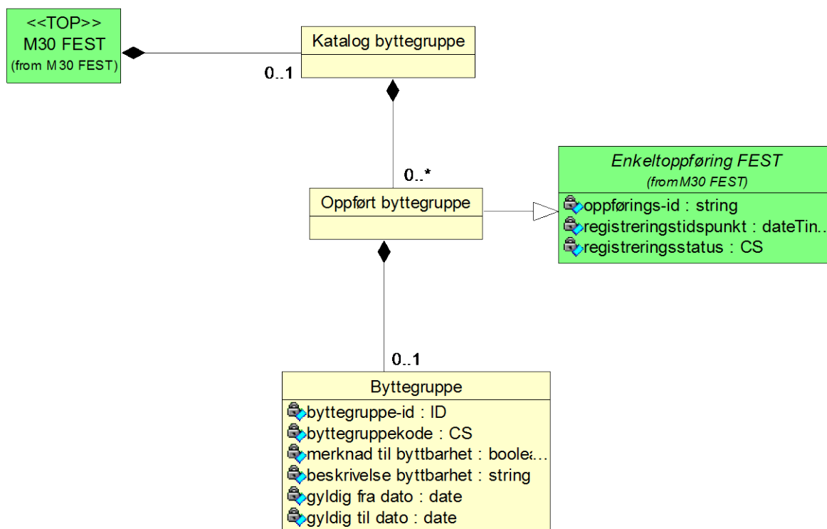
Diagram: Byttegruppe
